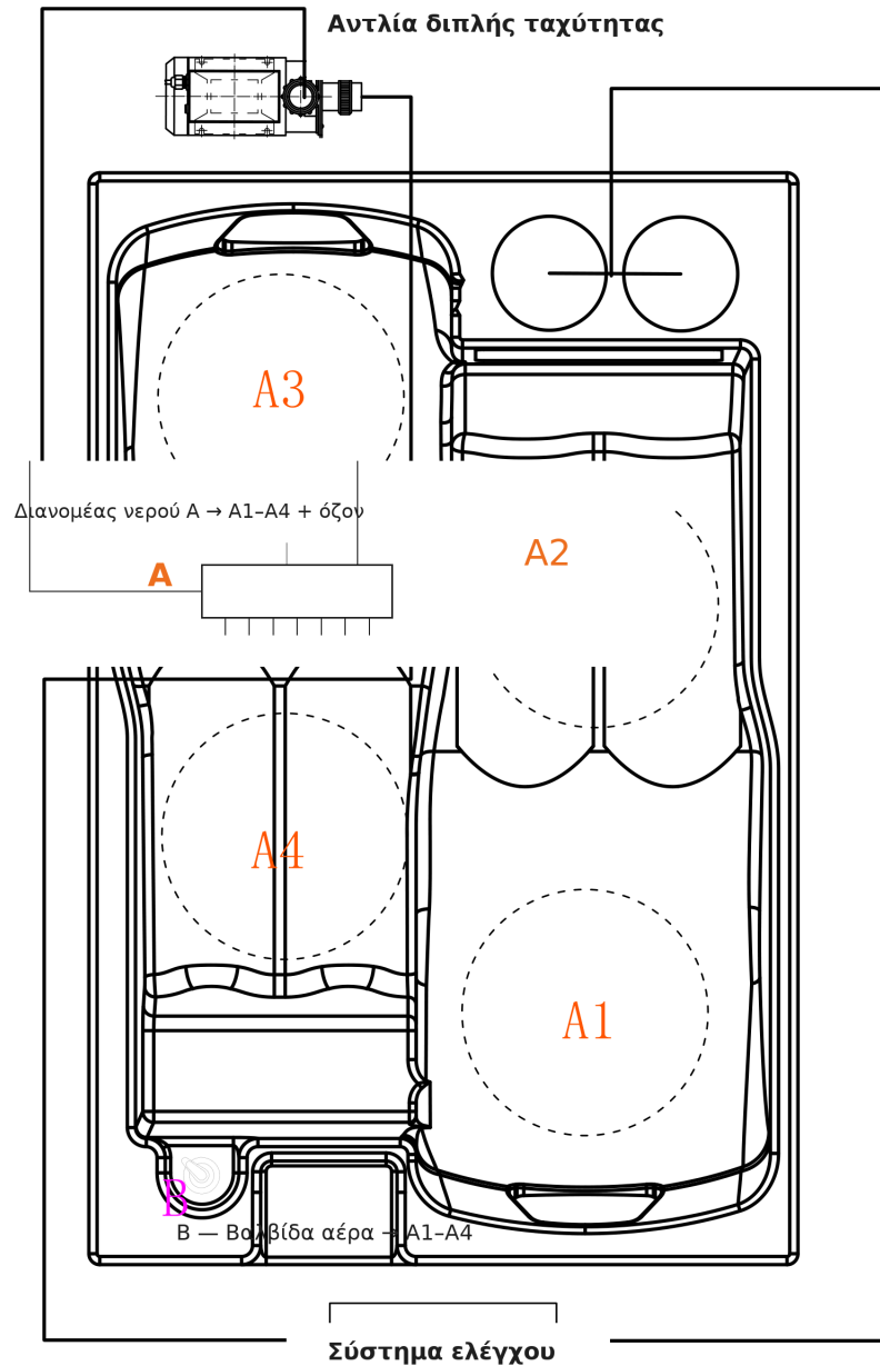
Σχήμα 2 — Διάταξη σωληνώσεων OX L303 (κάτοψη)
