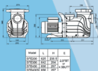
Dimensions
