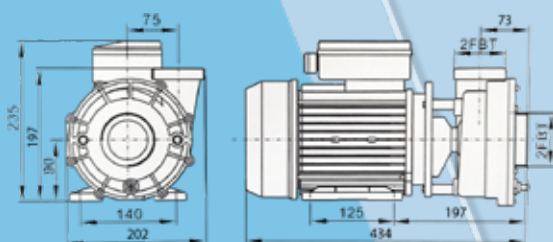
Dimensions
