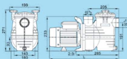
Dimensions
