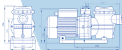
Dimensions
